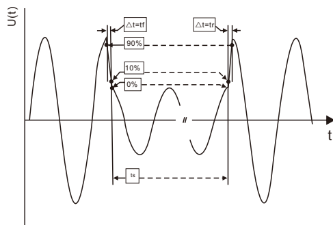
电压中断示意图
