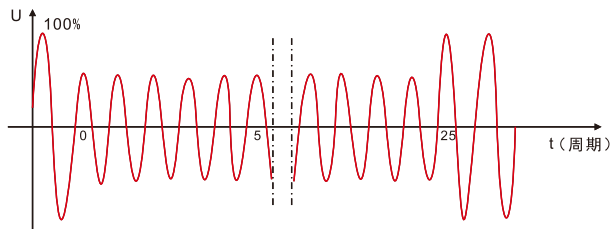
电压变化示意图
